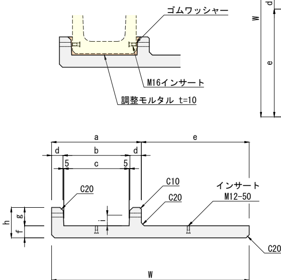
接続詳細図
