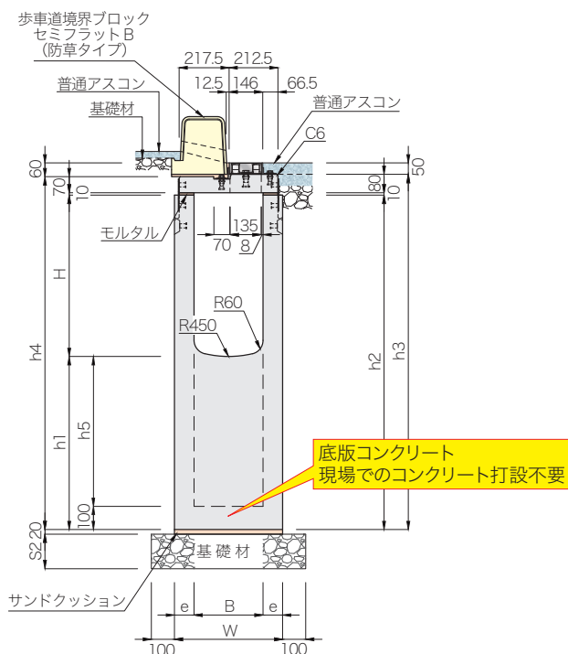
布設標準構造図(参考)
