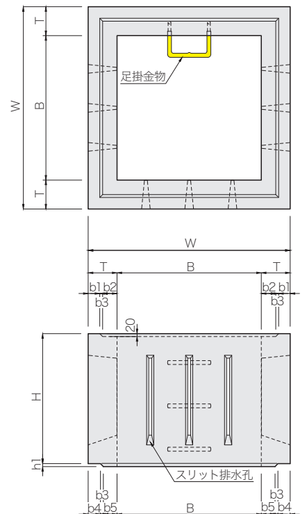
TYS大型浸透柵1000 浸透側塊 規格寸法表
