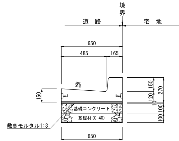
A135° コーナー右
