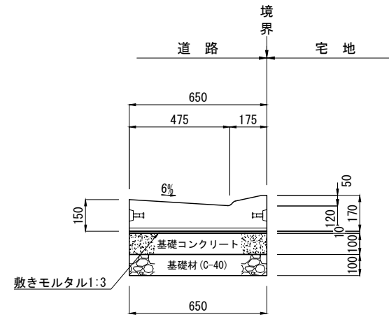
AD90° コーナー右
