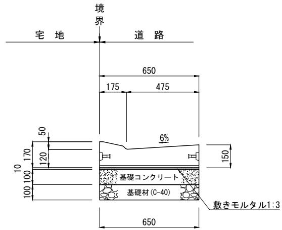
AD90° コーナー左
