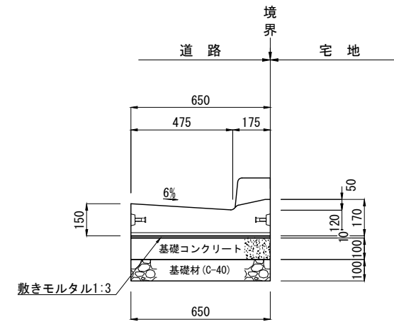
A斜135° コーナー右 (右下がり)
