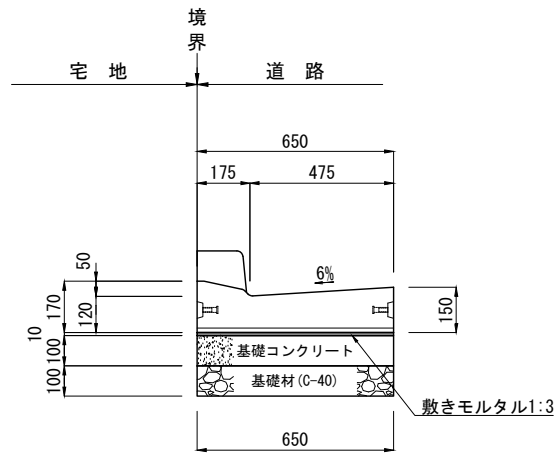
A斜135° コーナー左 (左下がり)
