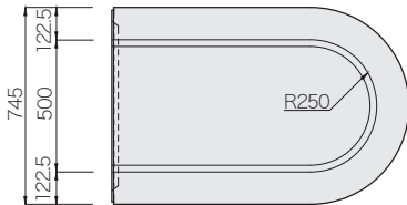
端末(シフト一体型) 参考質量 :525kg (注)仕入れ品対応です。
