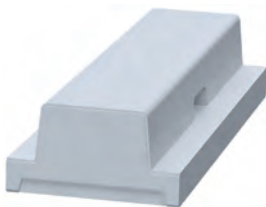
端末(シフト一体型) 参考質量 :525kg (注)仕入れ品対応です。
