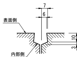
目地詳細図
