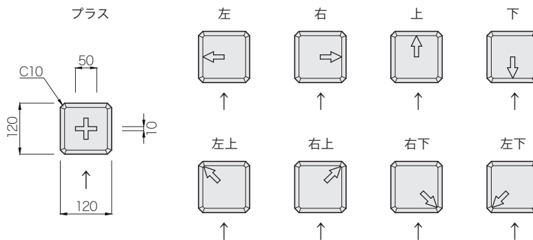
平面図 (杭頭矢印の種類)
