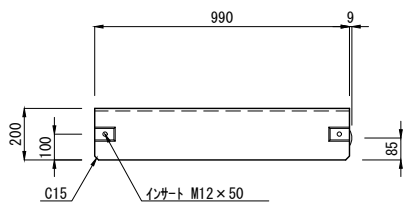
B低 H=20 L=1000 (参考質量：305kg)
