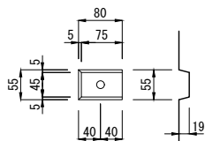
ジョイント部詳細図
