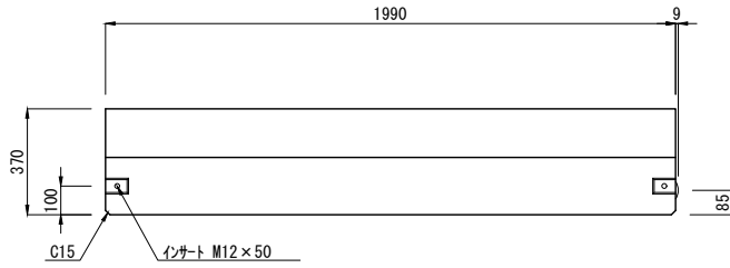
B基本 L=2000 (参考質量: 769kg)
