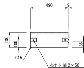
B低 H=20 L=500 (参考質量：152kg)
