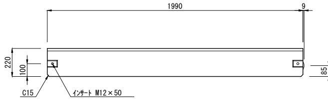
BD低 L=2000 (参考質量：629kg)
