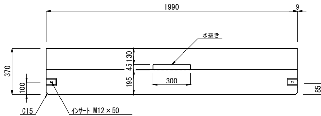
B水抜き L=2000 (参考質量: 762kg)
