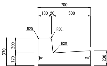
BD斜左 L=1000 (参考質量: 361kg)
