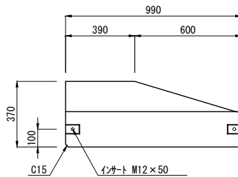
B斜左 H=20 L=1000 (参考質量：358kg) (注)斜右は斜左と左右対称
