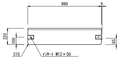
B斜左 H=20 L=1000 (参考質量：358kg) (注)斜右は斜左と左右対称
