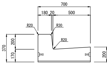
B斜左 H=20 L=1000 (参考質量：358kg) (注)斜右は斜左と左右対称
