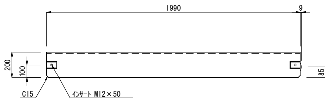
B低 H=20 L=2000 (参考質量：610kg)
