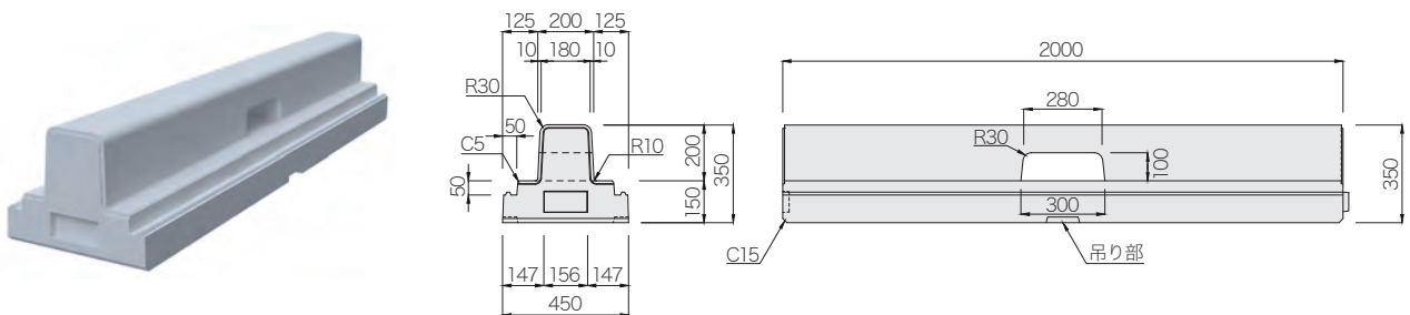
水抜き(防草) 参考質量 : 448kg
