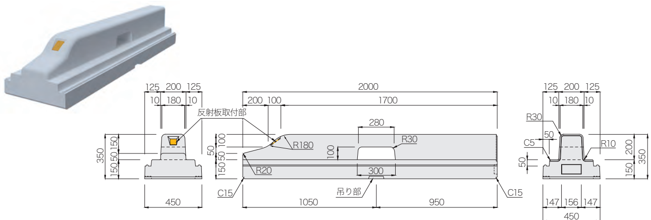
斜水抜き(防草)(反射板付き) 参考質量 : 434kg
