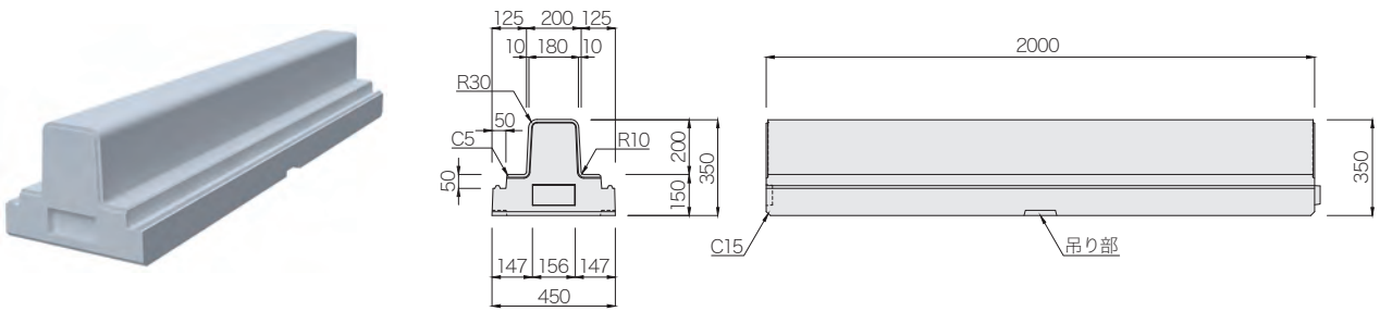
基本(防草) 参考質量 : 460kg
