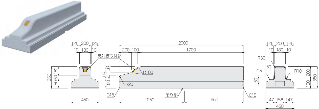
斜水抜き(防草)(反射板付き) 参考質量 : 434kg
