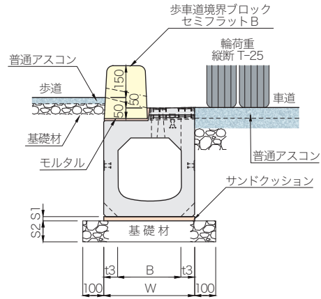
布設標準構造図(参考)
