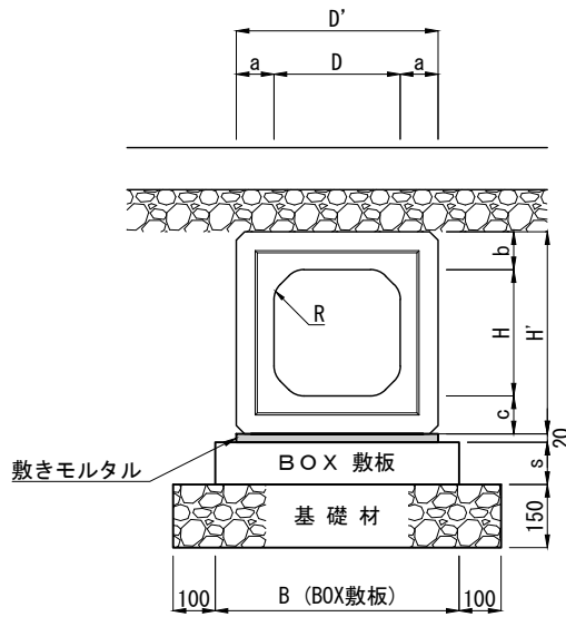
寸法表 [Y. T. C ボックスカルバート]
